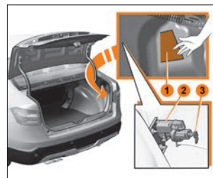
Рис. 7. Доступ к электроприводу (кузов «SE»)
