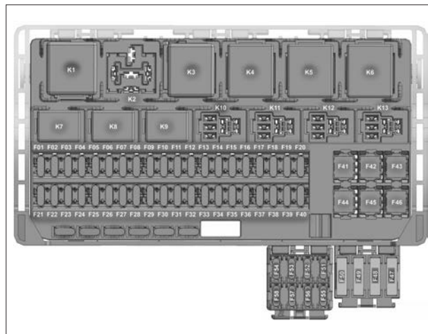
Рис. 3. Расположение предохранителей и реле в монтажном блоке салона
