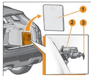
Рис. 6. Доступ к электроприводу (кузов «SW»)
