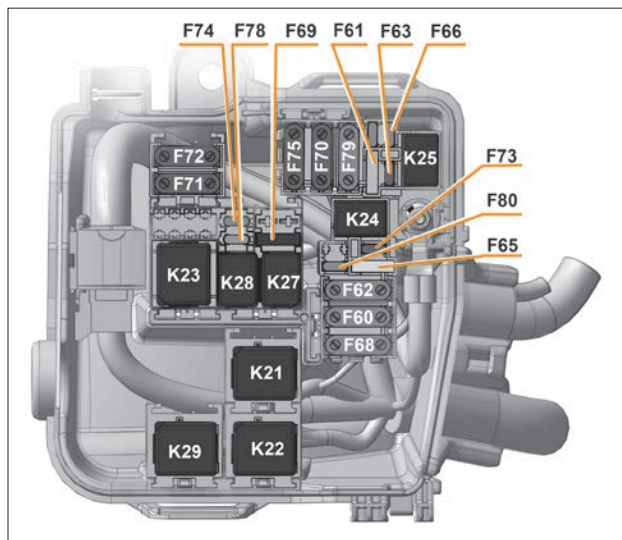
Рис. 1. Расположение предохранителей и реле в монтажном блоке моторного отсека
