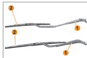
Рис. 8. Щетки стеклоочистителя
