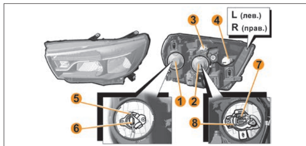
Рис. 11. Блок-фара
