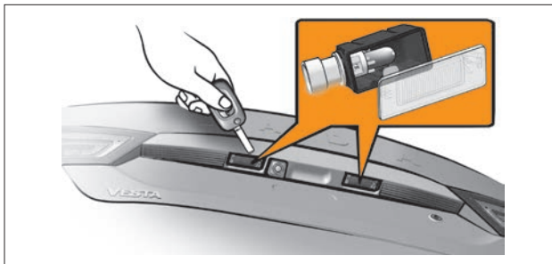
Рис. 18. Посадочное место фонаря освещения номерного знака
