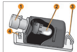
Рис. 17. Фонарь освещения номерного знака
