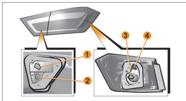
Рис. 13. Задние фонари
