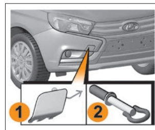
Рис. 9. Расположение передней буксирной проушины (в варианном исполнении)
