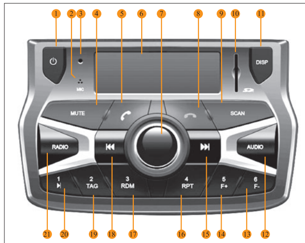
Рис. 1. Внешний вид и форма лицевой панели радиоприемника LADA Vesta
