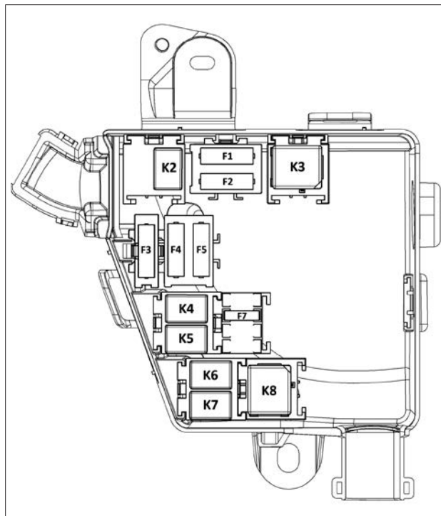
Рис. 3. Блок предохранителей и реле моторного отсека (ДВЦ K4M)
