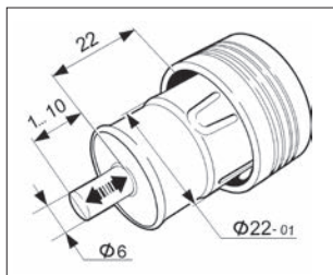
Рис. 21б. Размеры вилки электрического прибора для использования в патроне для исключения дополнительных потребителей
